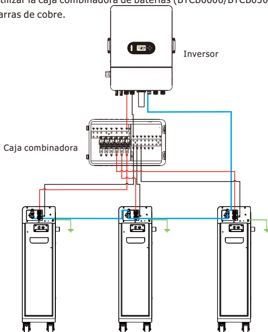
Figura 4-1 Conexión en paralelo de tres paquetes de baterías
