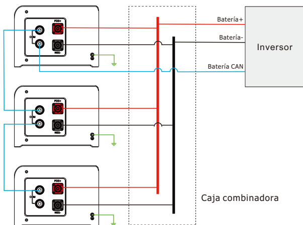
Figura 4-1 Conexión en paralelo de tres paquetes de baterías
