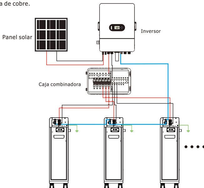
Figura 3-2 Diagrama de conexión de un sistema de baterías múltiples en
